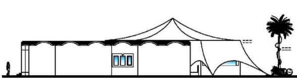
FACADE LATÉRALE Echelle 1/100
