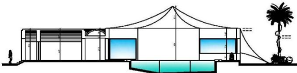
COUPE A-A Echelle 1/100
